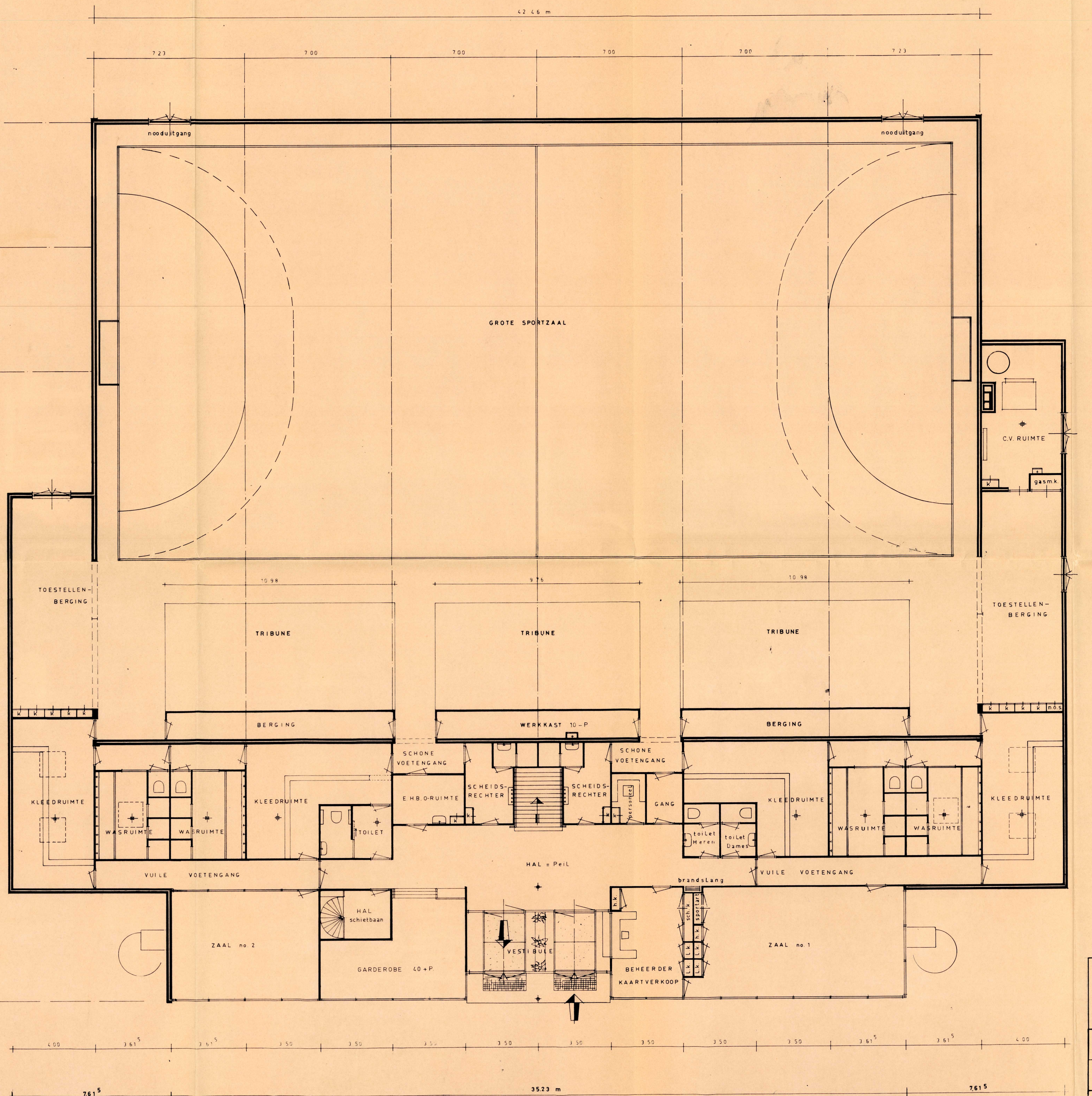
begane - grond
